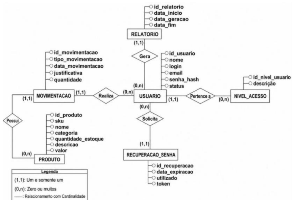
Figura 5 - Diagrama Entidade-Relacionamento (DER) Conceitual do Sistema Stock Master
