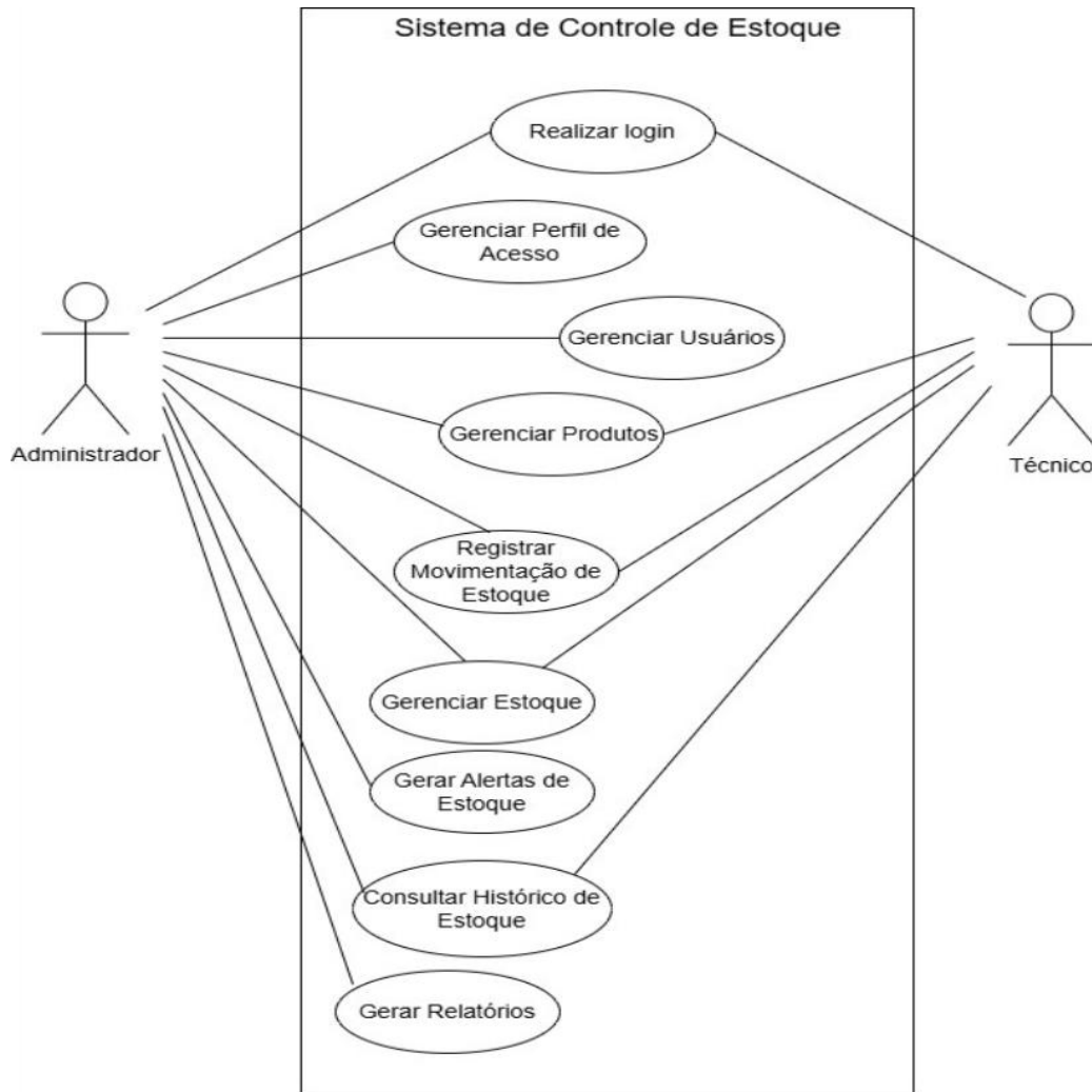
Figura 1 - Diagrama de Casos de Uso do Sistema Stock Master
