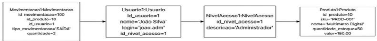
Figura 8 - Diagrama de Objeto
